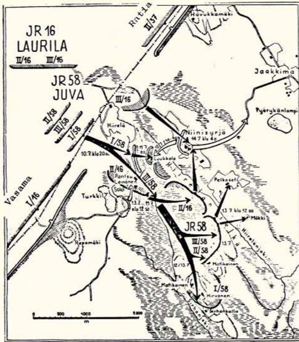
Kuva 3: 19. D:n hyökkäys 10.—13. 7.
