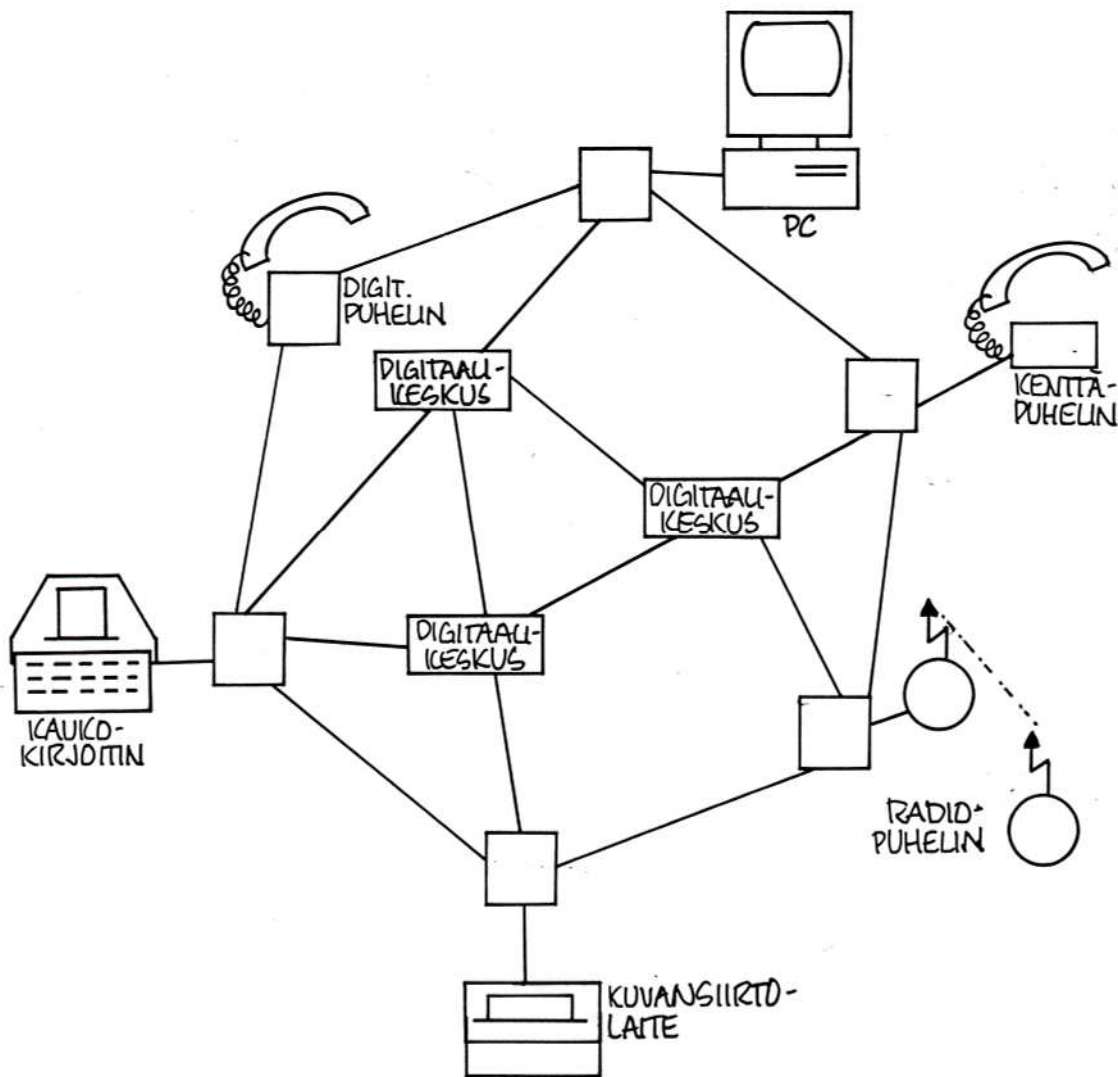
Integroidun verkoston periaate. Yhteydet voivat olla samoja kuin yllä, mutta niissä tieto on digitaalisessa muodossa eikä johto ole varattu pelkästään yhdelle päätelaitteelle kerrallaan.
