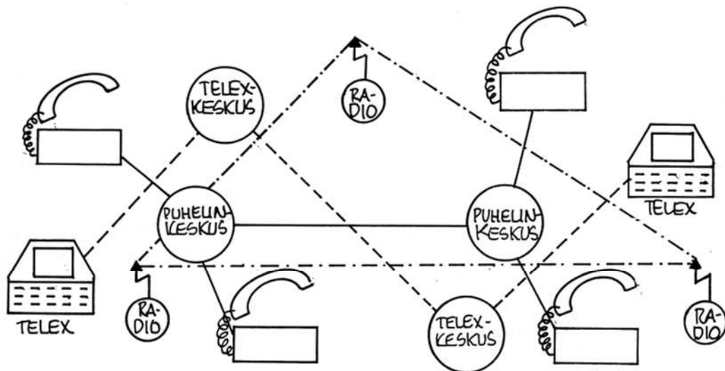
Perinteisen päällekkäisten verkkojen rakenteen periaate, joka vaatii runsaasti käyttöhenkilökuntaa ja on haavoittuva.
