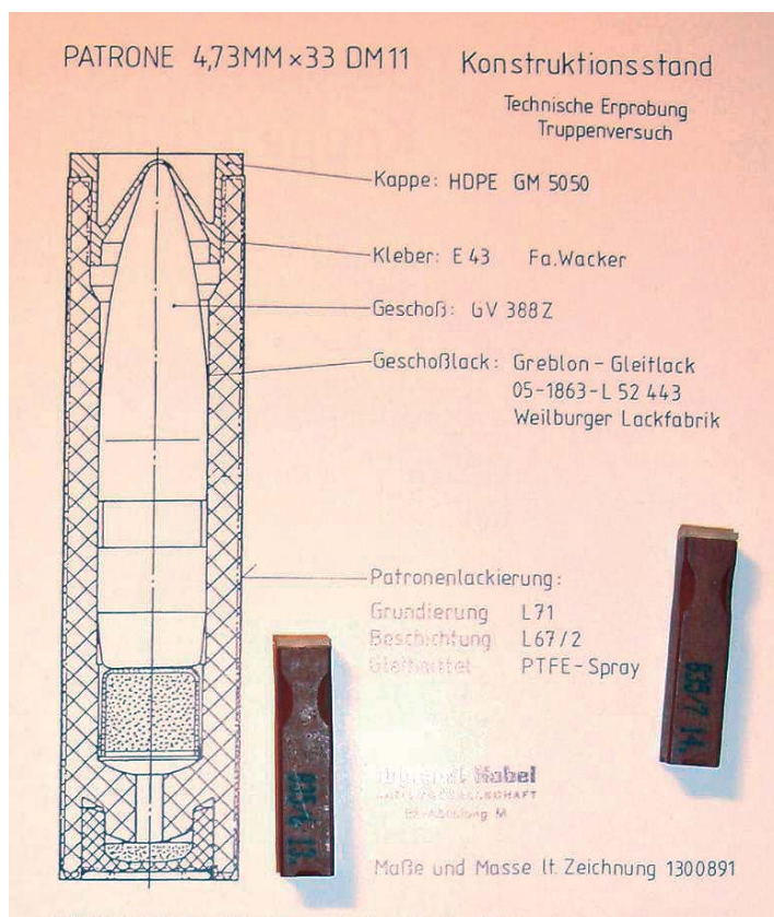
DM11 patruuna Saksalaisen valmistajan piirroksen verrattuna.
