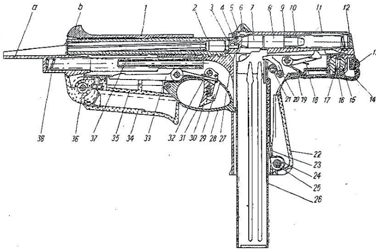
Rys. 0. Przekrój 9 mm pistoletu maszynowego wz. 1963:
