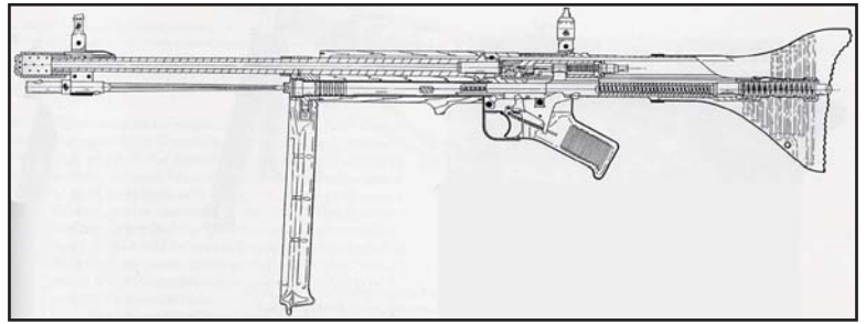
Läpileikkauspiirros FG42 malli E kivääristä, jossa etuet käännetty käyttöasentoon. Huomaa hyvin suoraviivainen rakenne, jossa asepiipun keskiakseli asettuu samalle linjalle ampujan olkatuennan kanssa vähentäen merkittävästi rekylin piipun suuta nostavaa vaikutusta.
